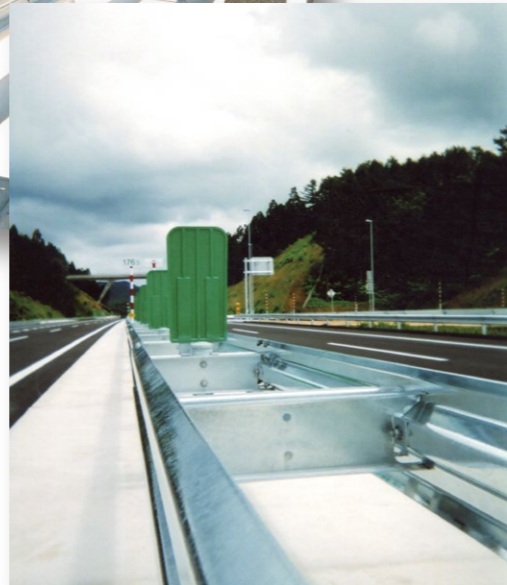
Asタイプ、 カラー：グリーン
